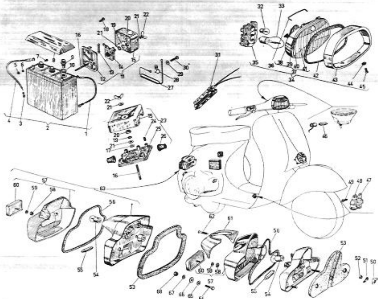
GRUPO EQUIPO ELECTRICO: Faro delantero (S 64)-Batería y Rectificador (S 61)-Rectificador (S 64: 100001 + 123500) Caja bornas y Rectificador (S 64: 123501 en adelante)-Caja bornas (N 64: 211802 en adelante, L 64: 211802 en adelante)-Piloto 150 "5" e Interruptor "Stop" (S 61 y S 64)
