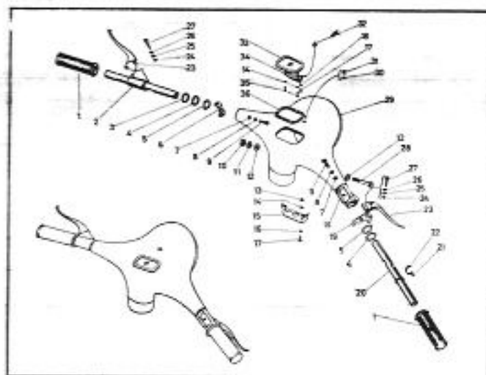
GRUPO DIRECCION-SUSPENSION
