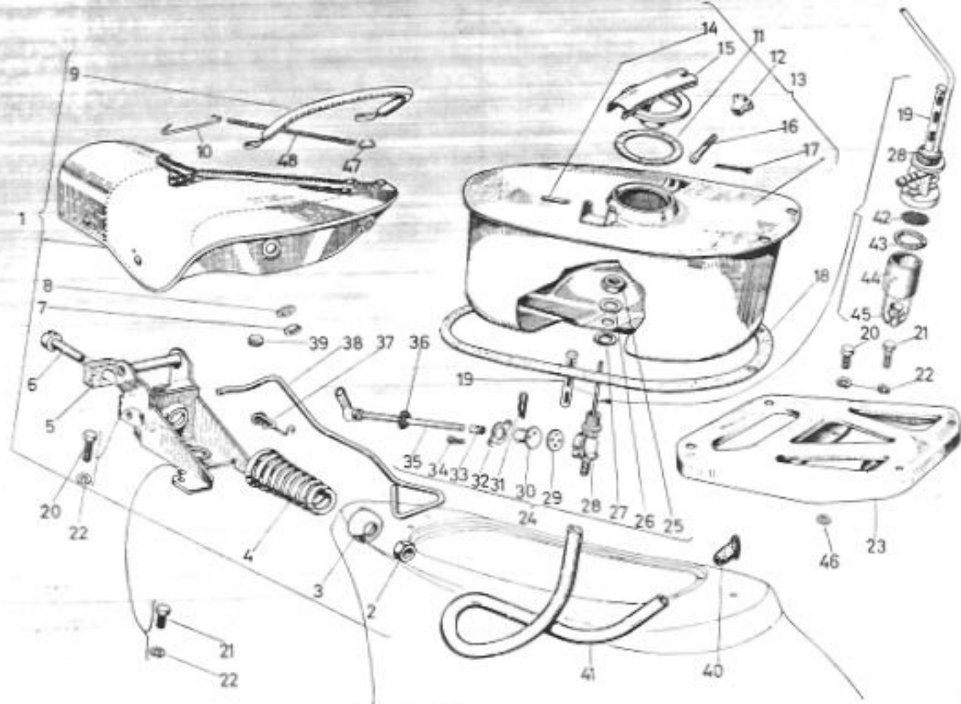
GRUPO BASTIDOR: Sillín monoplexa (N 60 - N 61 - N 64) - Depósito y grifo gasolina (N 60 - S 60 - N 61 - S 61 - 1L 62 - F 62 - 2L 62 - N 64 - L 64 - S 64) - Portacapijales (N 60 - N 61 - N 64).
