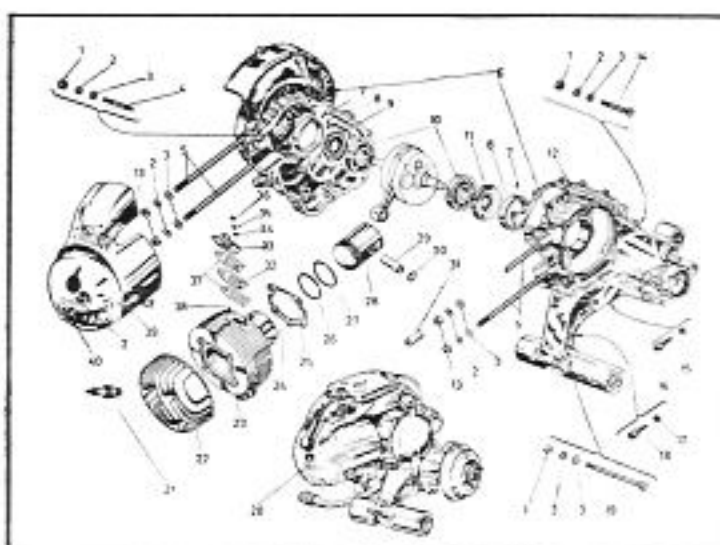
GRUPO MOTOR
