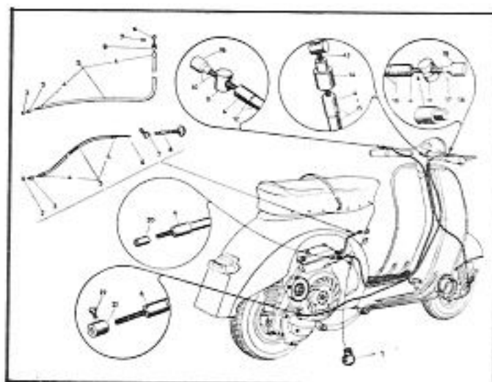
GRUPO TRANSMISIONES
