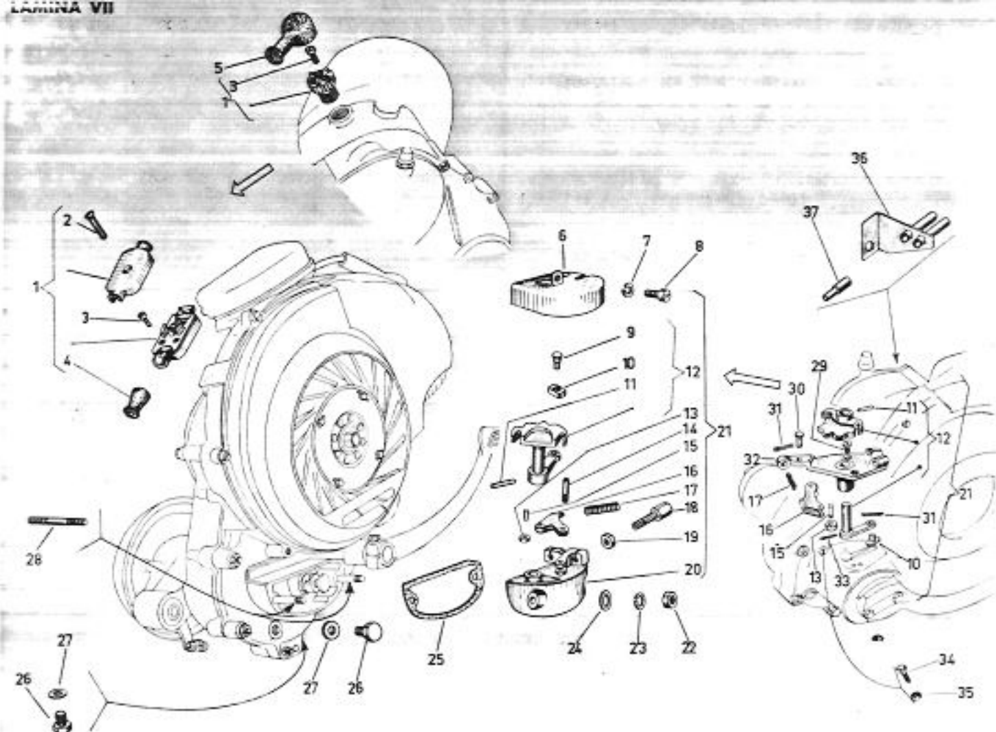
GRUPO MOTOR: Selector cambio (todos) - Toma B. T. (todos excepto: N y L 64 desde el chasis n.º 211802, S 64 desde el chasis n.º 123501).
