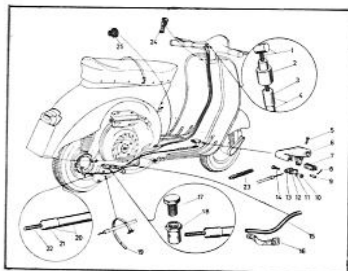
GRUPO TRANSMISIONES
