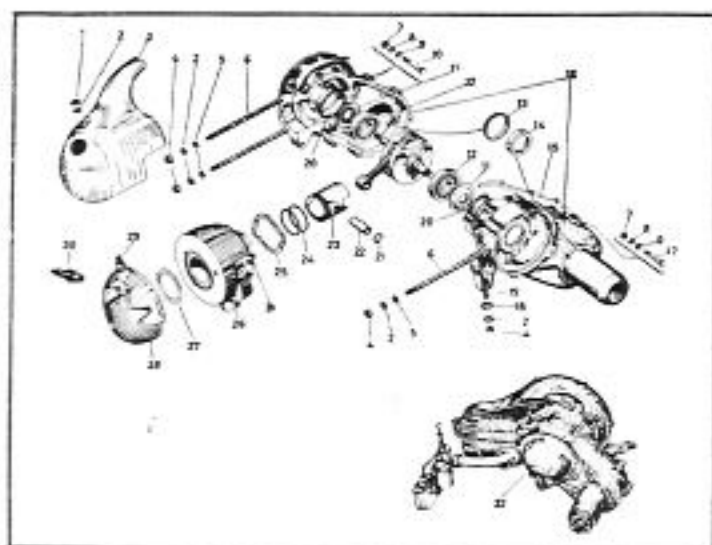
GRUPO MOTOR
